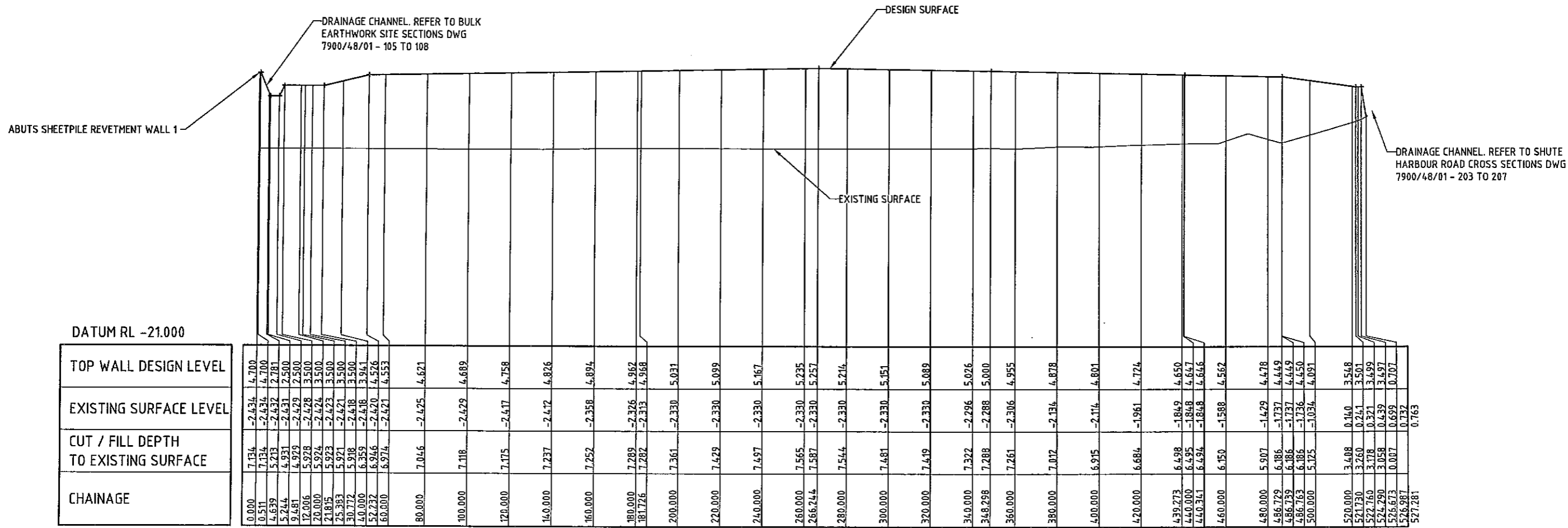
WALL 3 - BUND WALL LONGITUDINAL SECTION SCALE: HORIZONTAL - 1:1000 VERTICAL - 1:200
